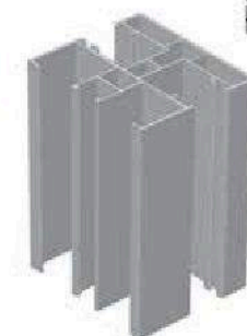
Coulisse PVC 60x52x60 mm (sans brosse) GL611-01
