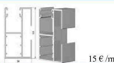
Coulisse alu 53x34x53 mm (sans brosse) GL311
