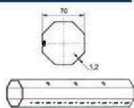
Axe acier octogonal AX70B15-52
