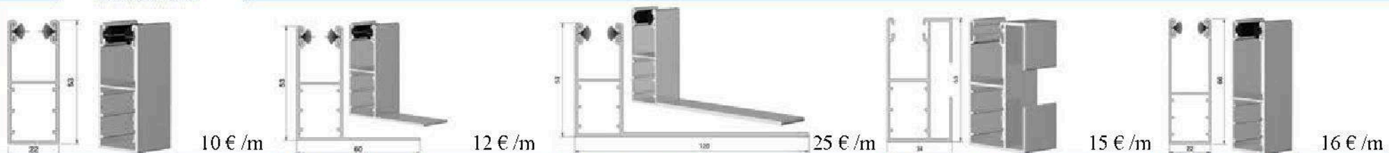
Coulisse alu 53x22x53 mm sans aile GL100
