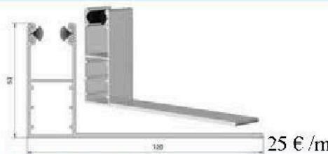
Coulisse alu 53x120x53 mm avec aile 120 mm GL112
